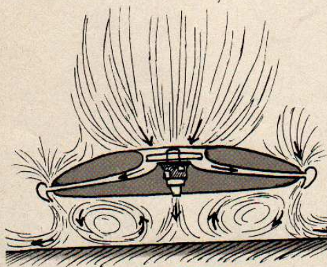
Aérodyné AVRO VZ 9V. Écoulement au voisinage du sol
