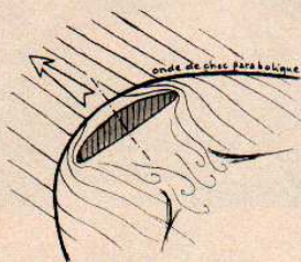
Aérodynne lenticulaire en déplacement supersonique
