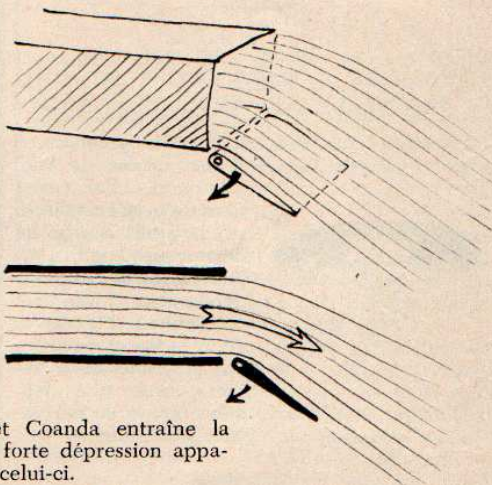
Décollement du jet
