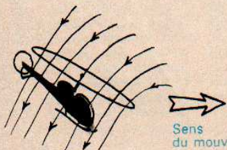
Vol en translation
